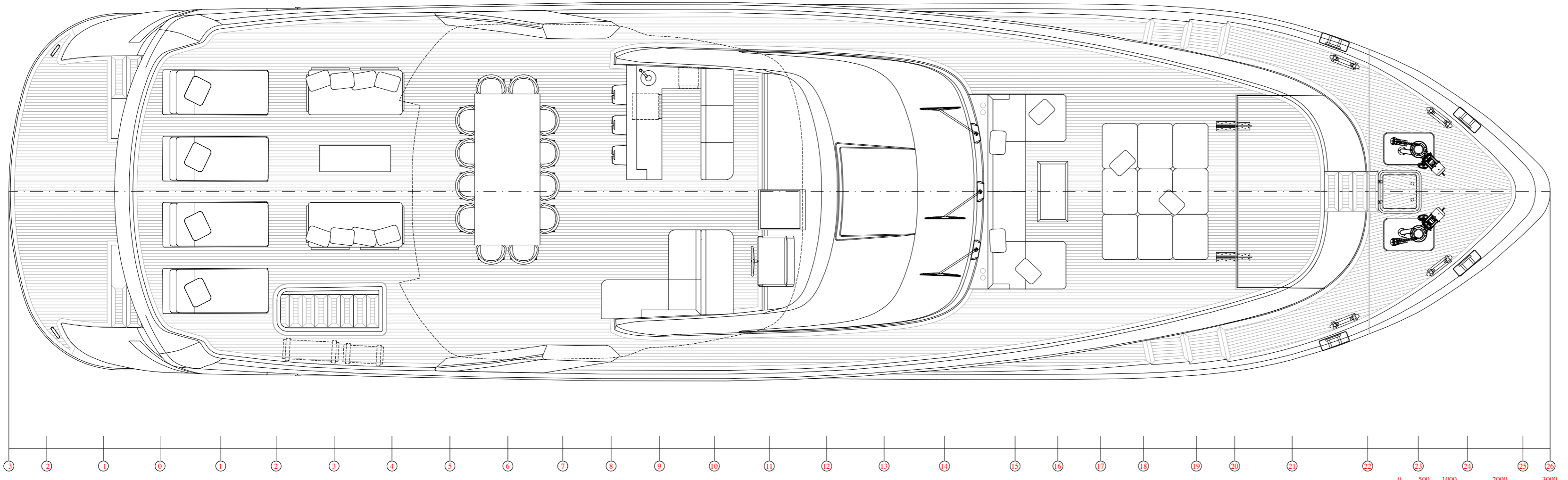
SUNDECK SCALA METRICA
