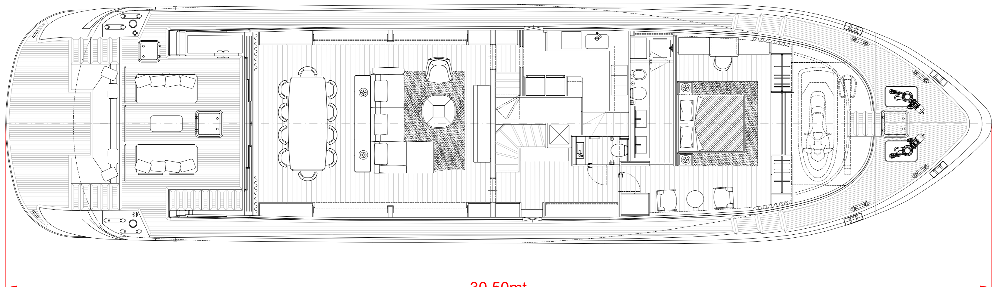
MAINDECK SCALA METRICA
